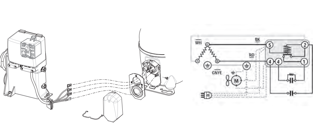
SM10 - NE CSR Box
